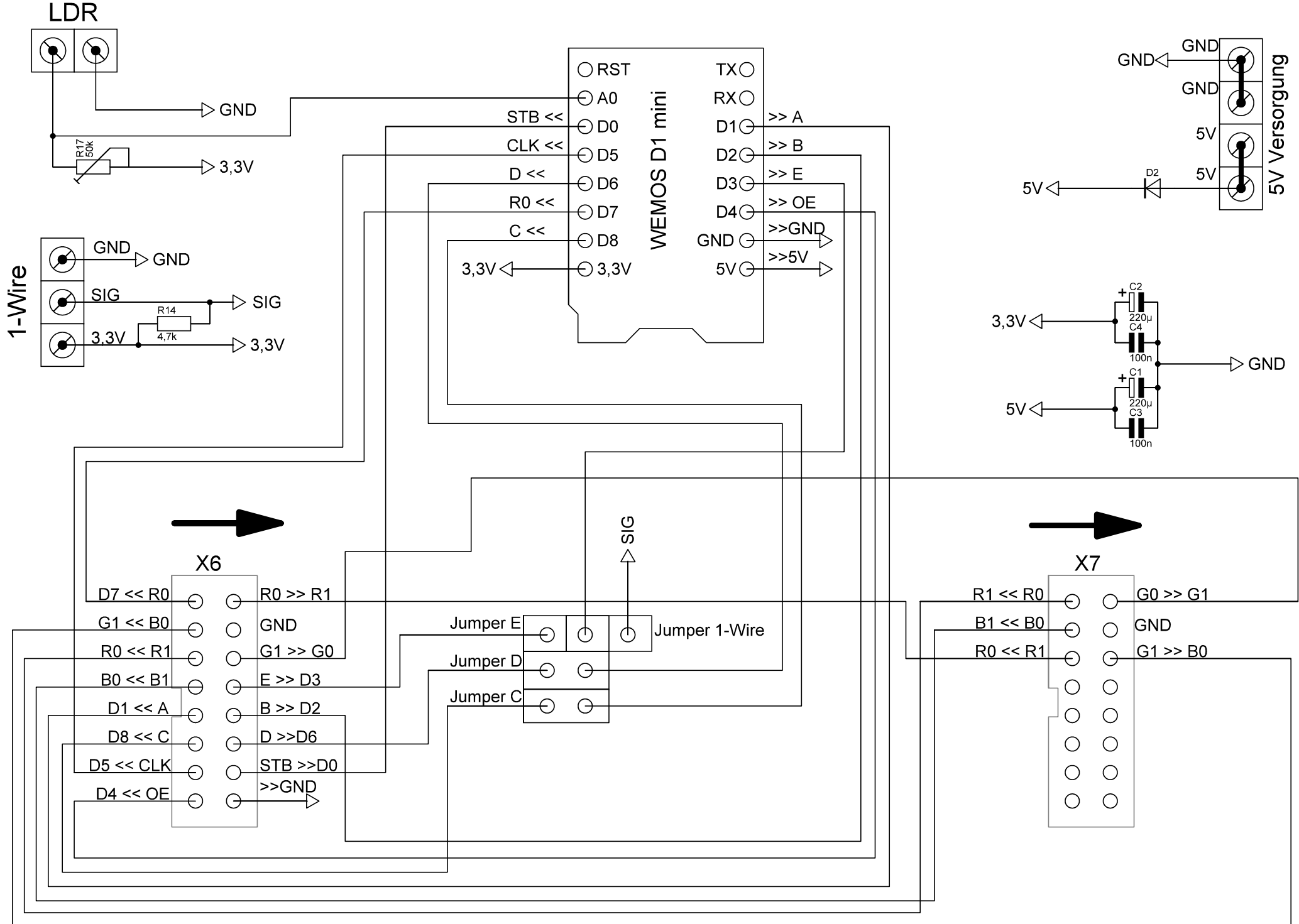
X6: Verbindung mit Display zum direkten Aufstecken
