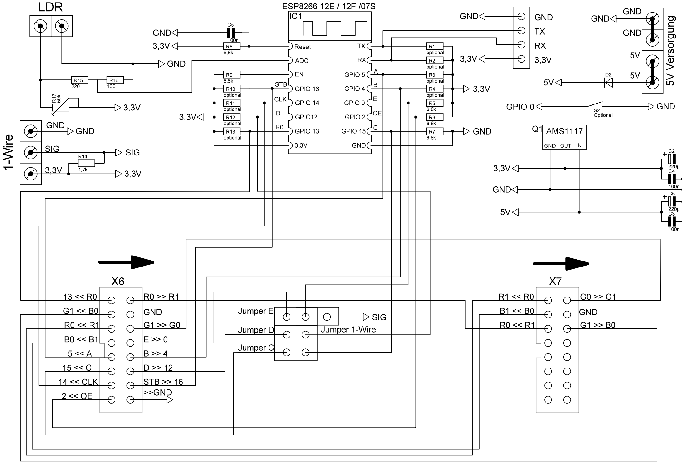
X6: Verbindung mit Display zum direkten Aufstecken
